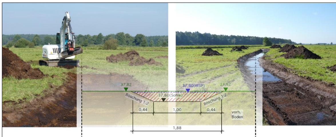
Abb. 3: Profilierung der Trasse, die das Wasser in die Vernässungsfläche bringen soll nach Vorgaben (hier Profilquerschnitt) der Ausführungsplanung
